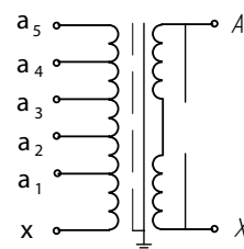
Рис. 2. Принципиальная электрическая схема трансформаторов ОЛ-2,5 и ОЛ-4
