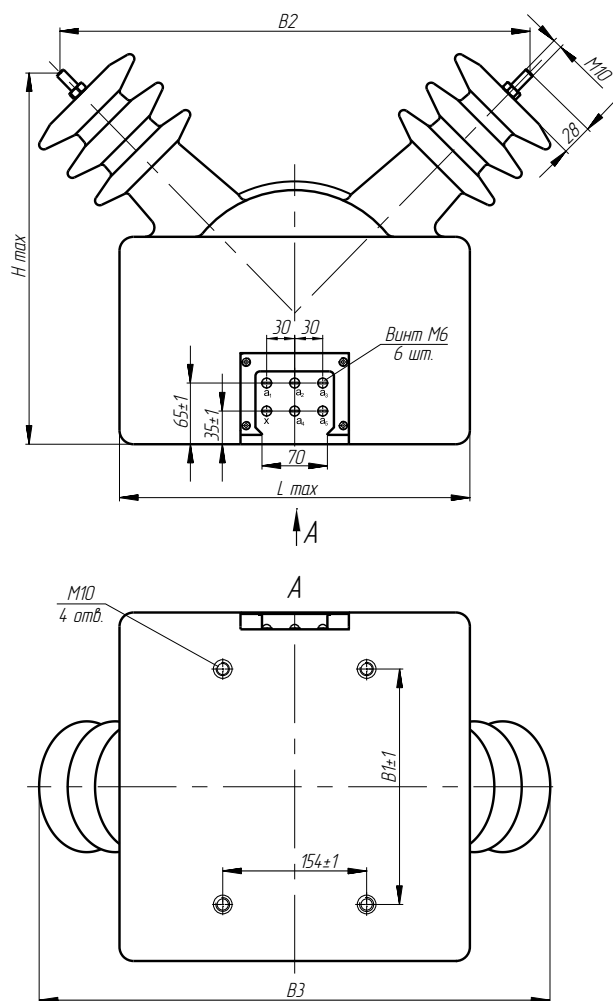
Рис. 1. Общий вид трансформаторов ОЛ-2,5 и ОЛ-4
